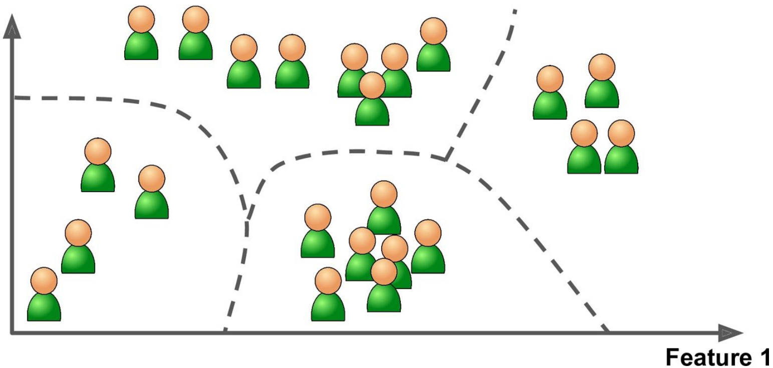
Figure 1-8. Clustering
